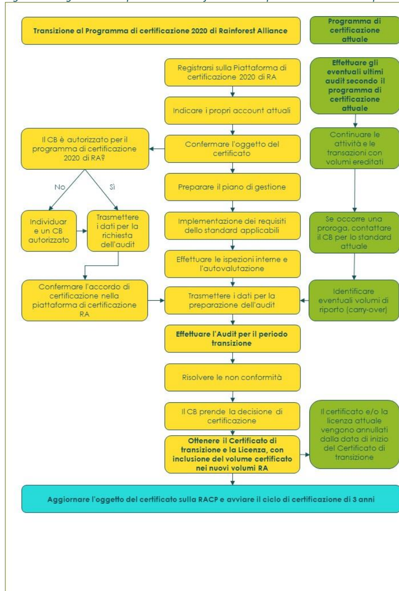
Figura 1: Diagramma del processo di certificazione nel periodo di transizione per i CHs agricoli in transizione
