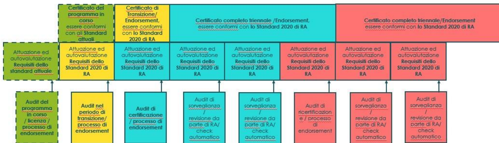
Figura 16: Tempistiche di attuazione, ispezione, conformità e certificazione dei vari programmi durante il periodo di transizione ed oltre.
