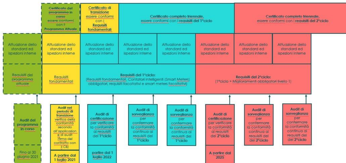
Figura 3: Tempistiche di attuazione, ispezione, conformità e certificazione dei vari programmi durante il periodo di transizione ed oltre.
