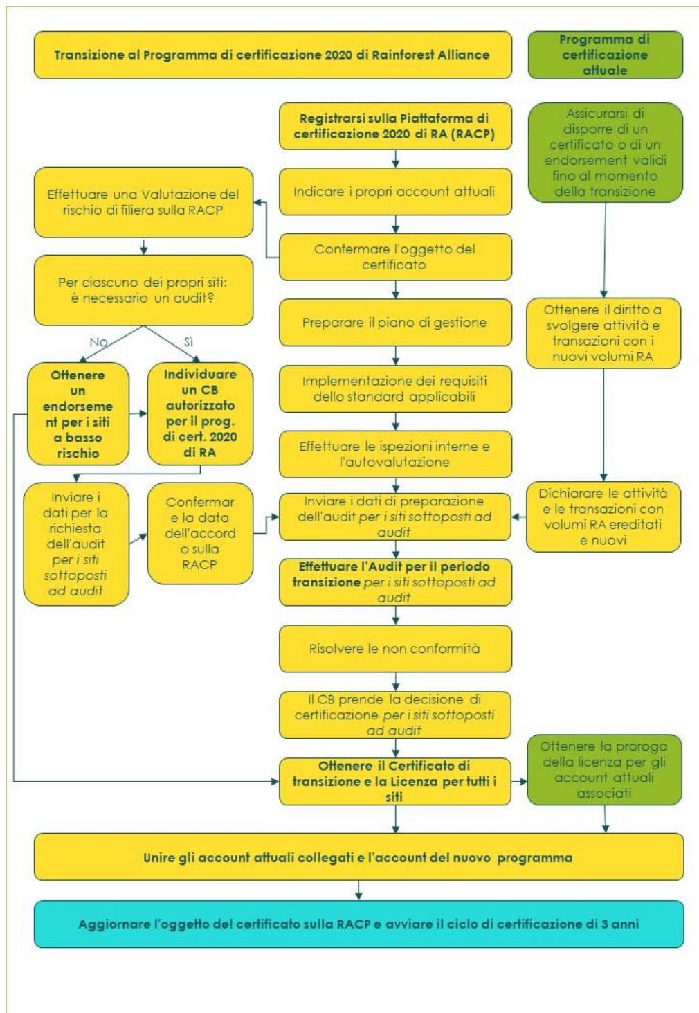
Figura 14: Diagramma del processo di certificazione nel Periodo di Transizione per i CHs di filiera in transizione.
